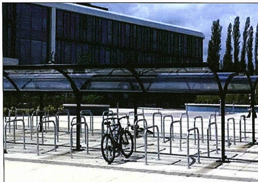
Figur 5-3 Exempel på cykelparkering med väderskydd och ramlåsning. Källa: www.cykelboxen.se
